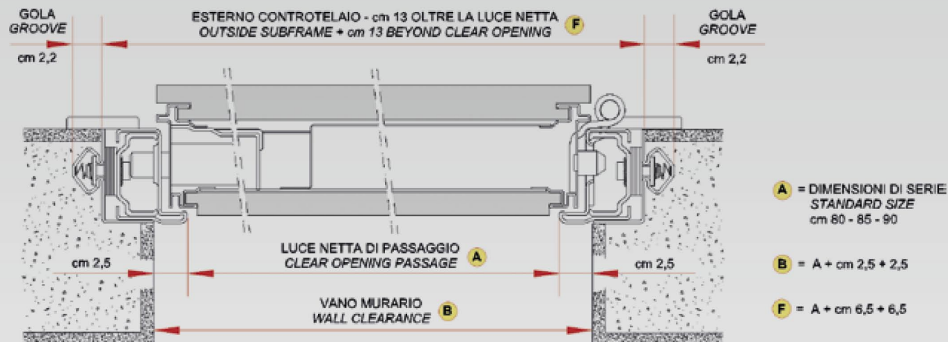
Porta 1 anta - Sezione orizzontale Single leaf door - Horizontal section
