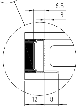
CANALINA ESTRUSA RIBASSATA CON ALETTA
