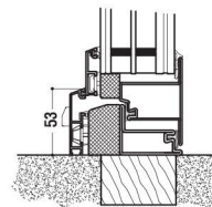
NODO INFERIORE LOWER NODE
